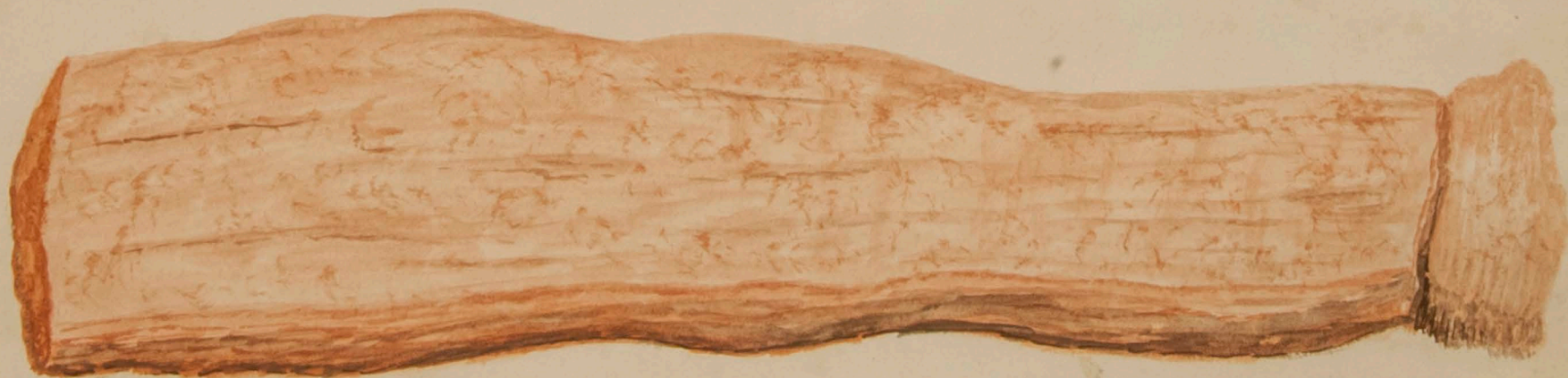
Otras piedras de El Yficernito.
