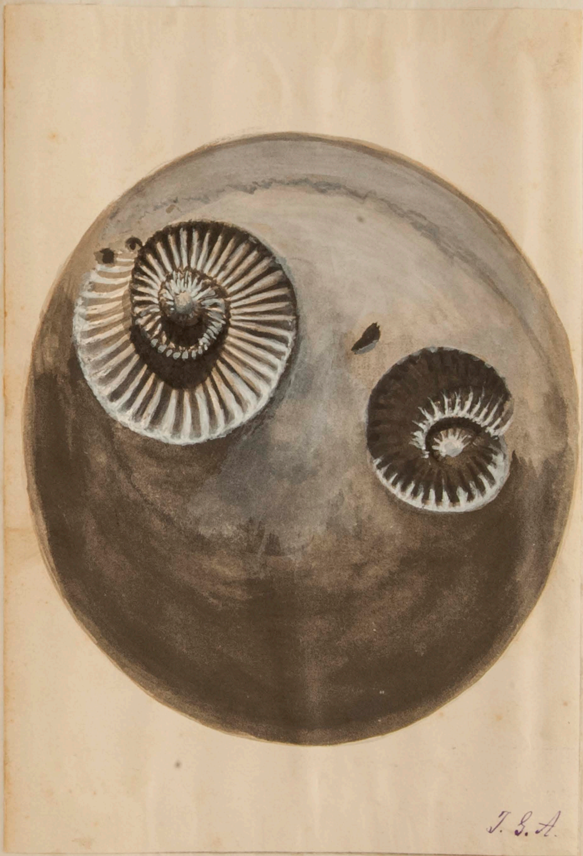
Ammonites fósiles impresas en cantos rodados de caliza carbonífera.
